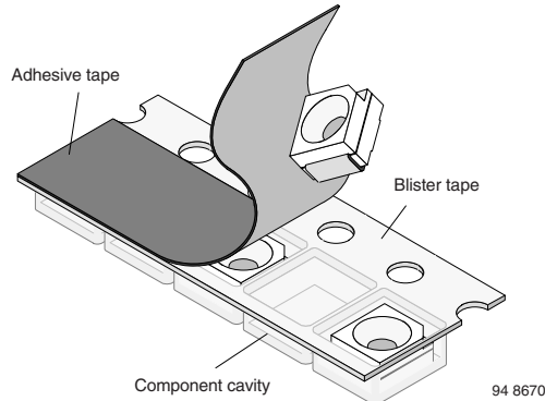
Fig. 10 - Blister Tape
