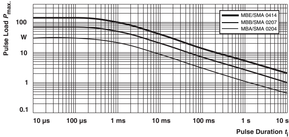
最大脉冲负载、单脉冲；运行 8000 小时后的允许的电阻变化
