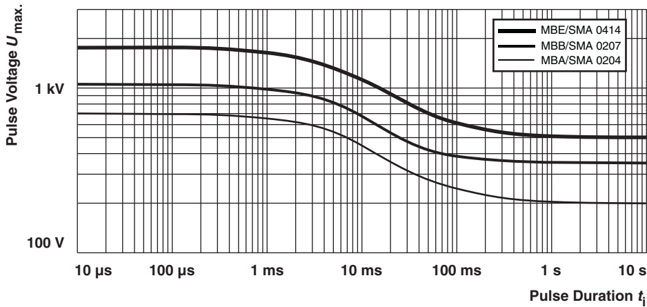
最大脉冲电压、单脉冲和连续脉冲；运行 8000 小时后的允许的电阻变化
