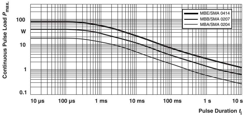
最大脉冲负载、连续脉冲；运行 8000 小时后的允许的电阻变化
