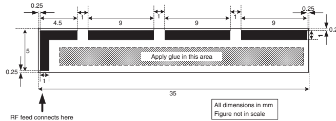
Fig. 5 - VJ 3505 Footprint
