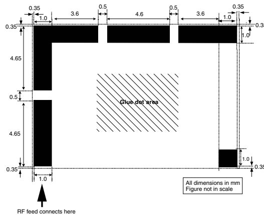
Fig. 6 - VJ 6040 Footprint
