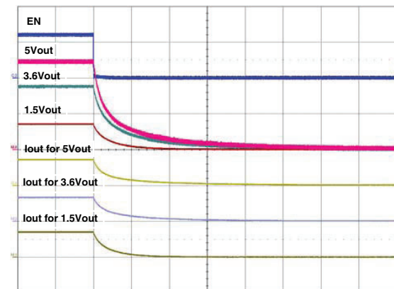
2 V/Div, 2 A/Div, 500 \mu s /Div
