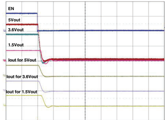
2 V/Div, 2 A/Div, 2 \mu s /Div
