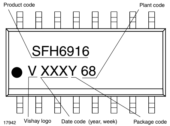
Fig. 10 - 16 Pin Miniflat
