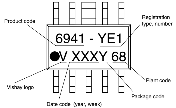
Fig. 4 - Minicoupler
