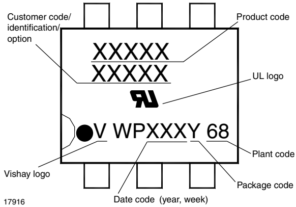
Fig. 1 - 6 Pin
