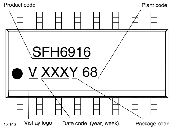
Fig. 10 - 16 Pin Miniflat
