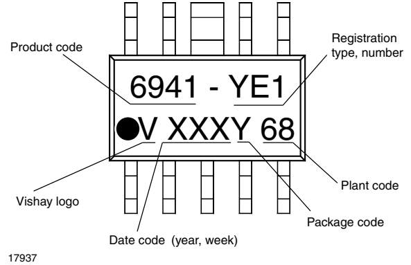
Fig. 4 - Minicoupler
