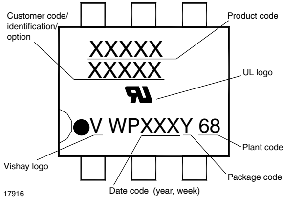
Fig. 1 - 6 Pin
