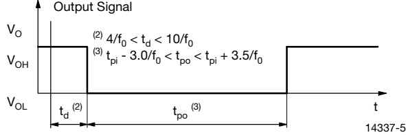
Fig. 1 - Output Function
