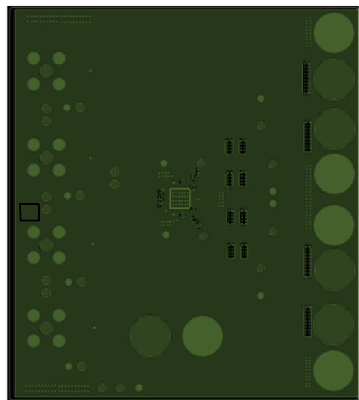
Fig. 24 - Inner 1
