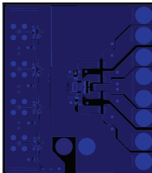
Fig. 26 - Bottom
