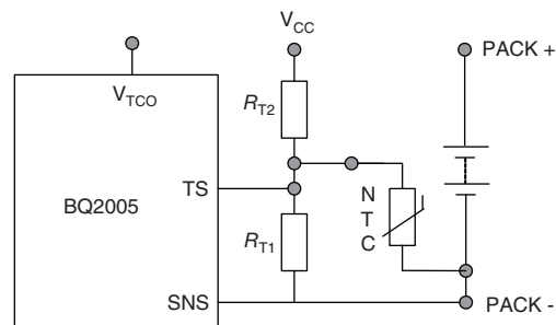
Fig. 20 - BQ2005
