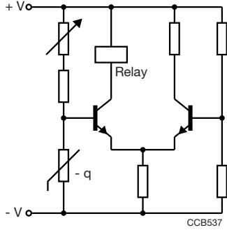
Fig. 16 - Simple thermostat
