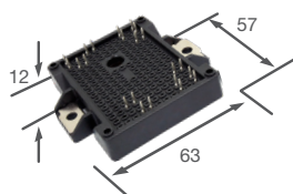
EMIPAK-2B
