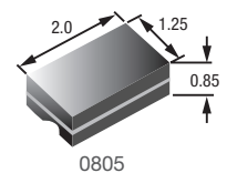
0805
