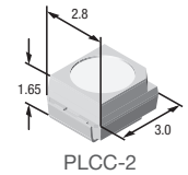
PLCC-2
