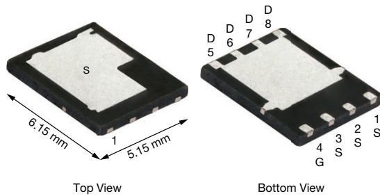
PowerPAK® SO-8DC
