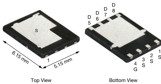
PowerPAK® SO-8DC
