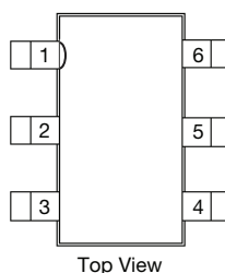
Fig. 3 - TSOT23-6 Package
