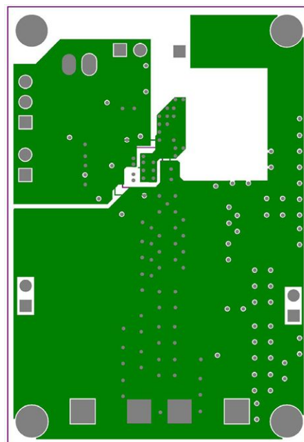
Fig. 22 - Inner Layer 2
