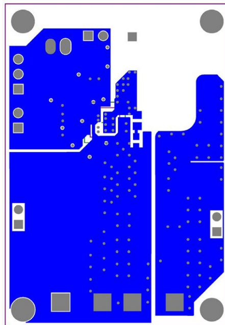
Fig. 23 - Bottom Layer
