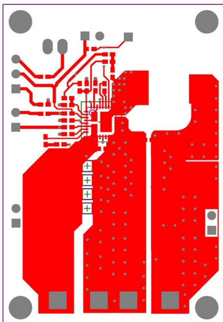
Fig. 20 - Top Layer
