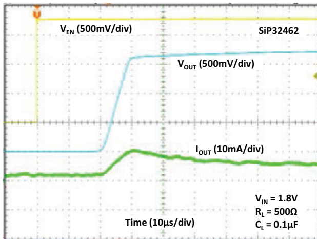
Fig. 28 - Turn-on Time
