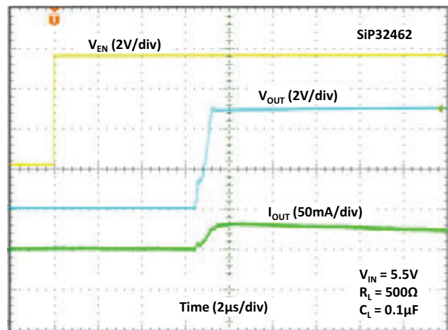
Fig. 31 - Turn-on Time
