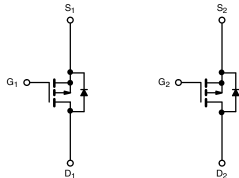
P-Channel MOSFET
