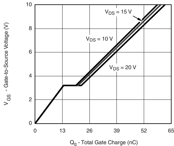
V_{DS} = 15\text{ V} V_{DS} = 10\text{ V} V_{DS} = 20\text{ V} Gate Charge
