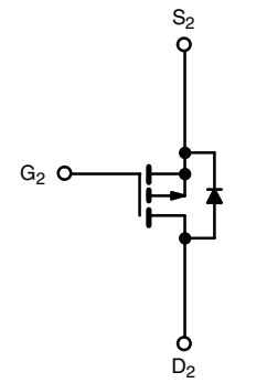
P-Channel MOSFET
