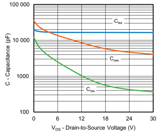
Fig. 4 - Capacitance
