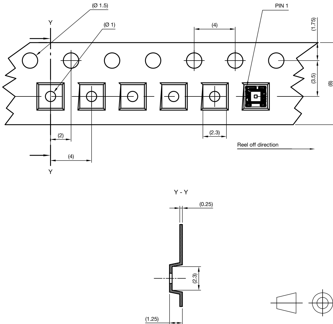
Fig. 13 - Taping
