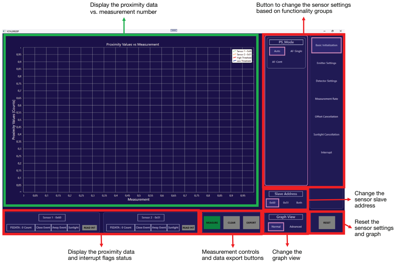
Fig. 2 - Demosoftware GUI
