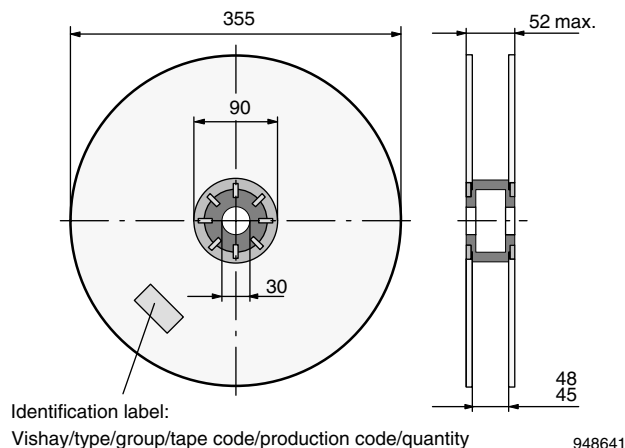
Fig. 16 - Reel Dimensions
