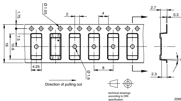
Fig. 21 - Tape Dimensions
