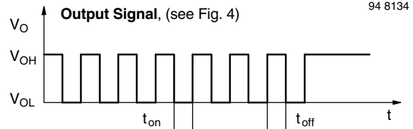
Fig. 3 - Output Function
