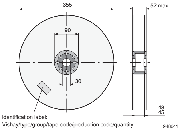
Fig. 7 - Reel Dimensions
