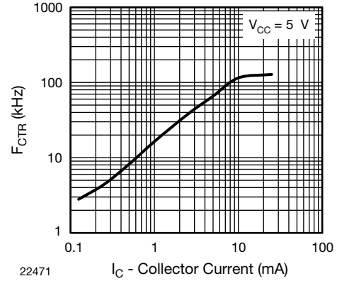
Fig. 12 - F_{CTR} vs. I_C
