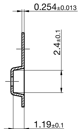
A-A Section
