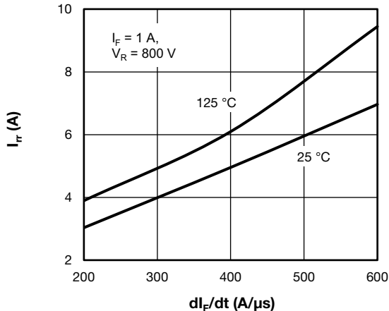
Fig. 8 - I_r (A) vs. dI_F/dt
