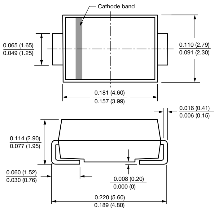
SMA-1 (DO-214AC)
