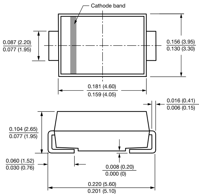
SMB-1 (DO-214AA)
